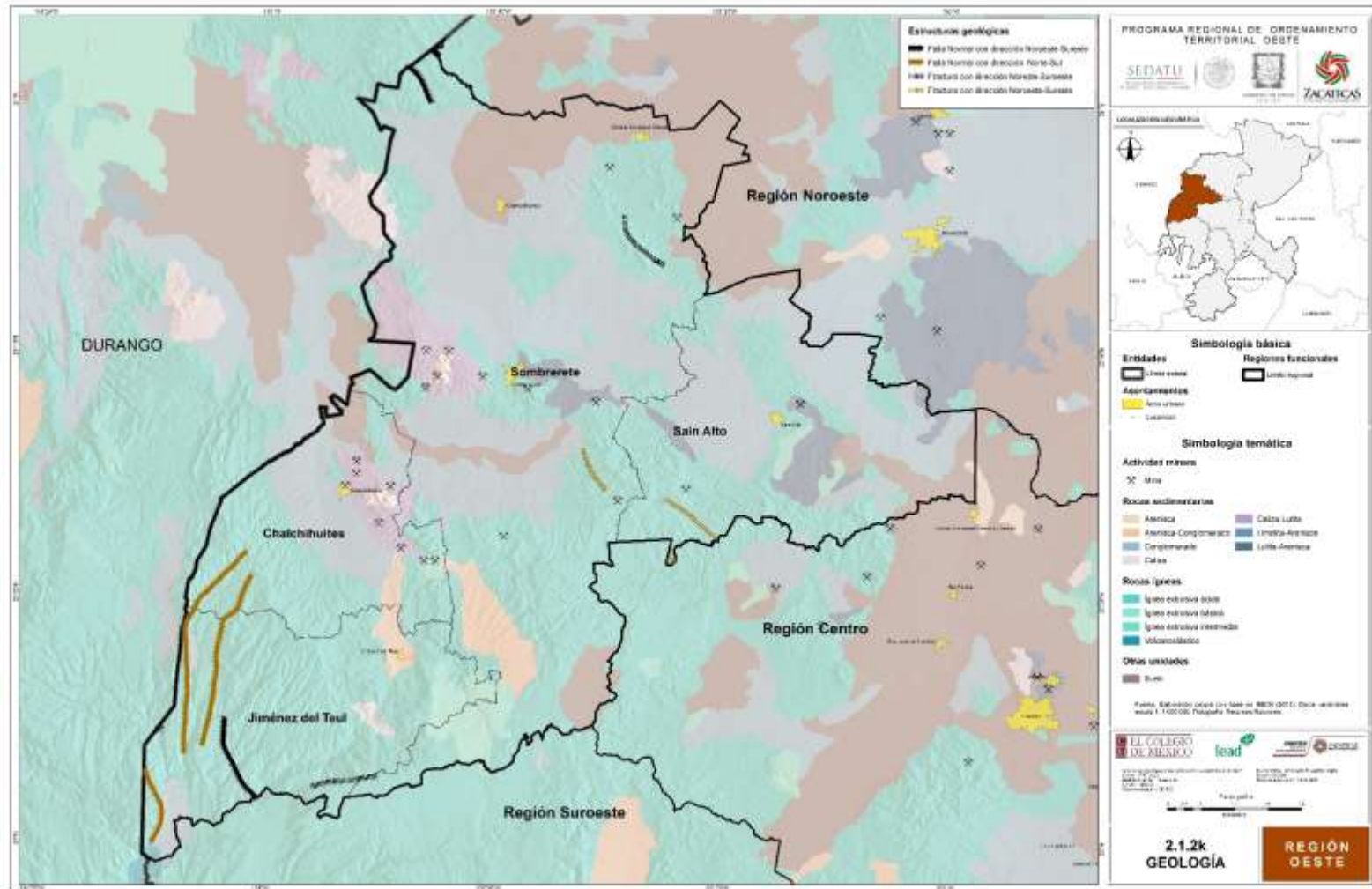
Mapa 2.1.2k. Geología
