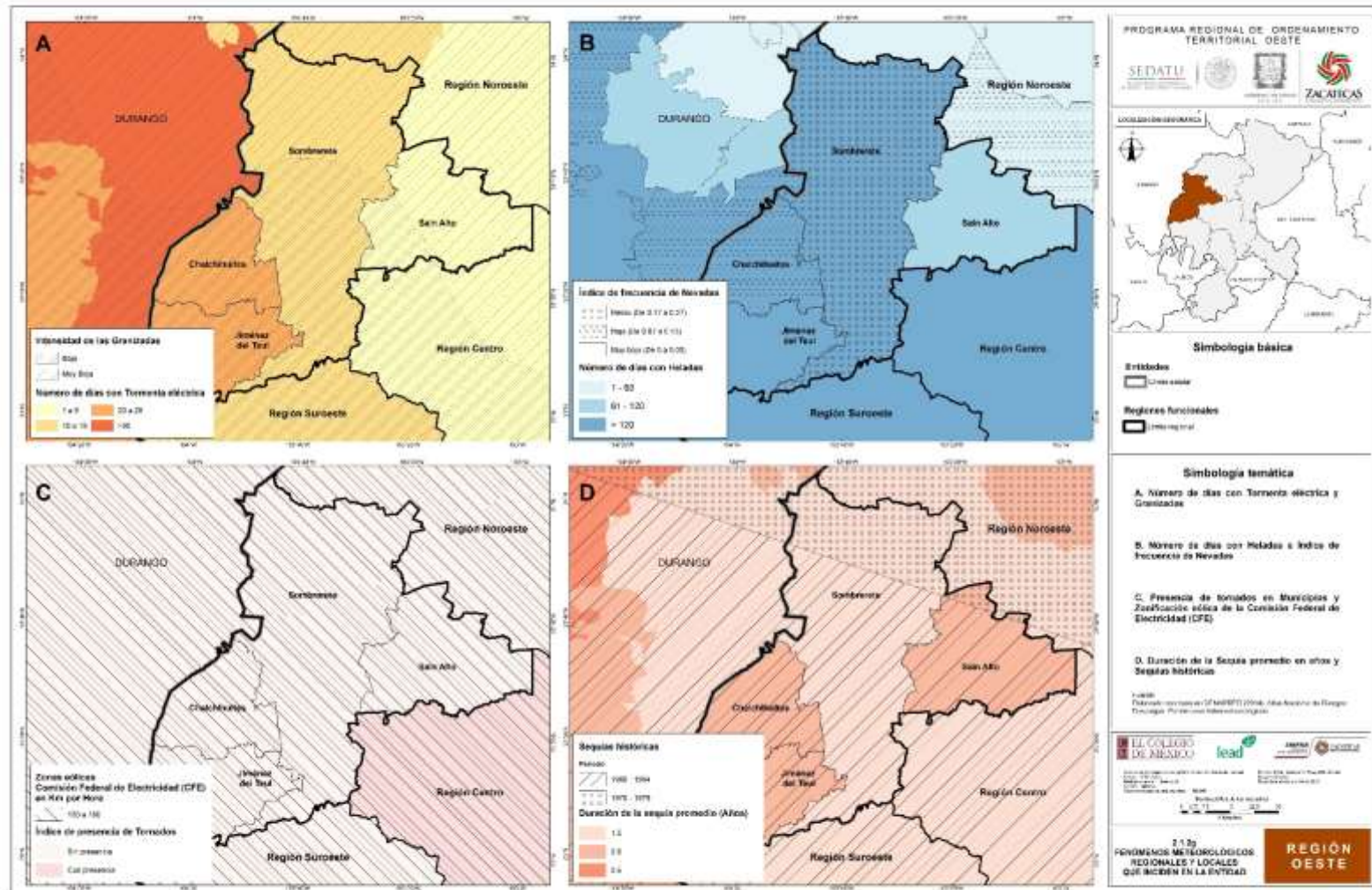
Mapa 2.1.2g. Fenómenos meteorológicos
