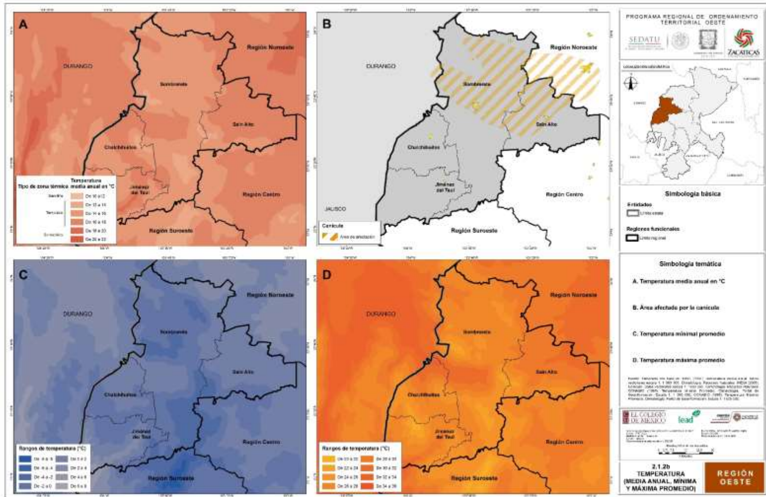
Mapa 2.1.2b. Temperatura
