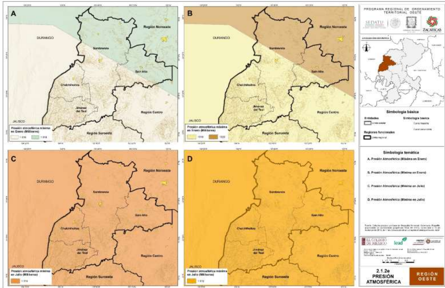
Mapa 2.1.2e. Presión atmosférica
